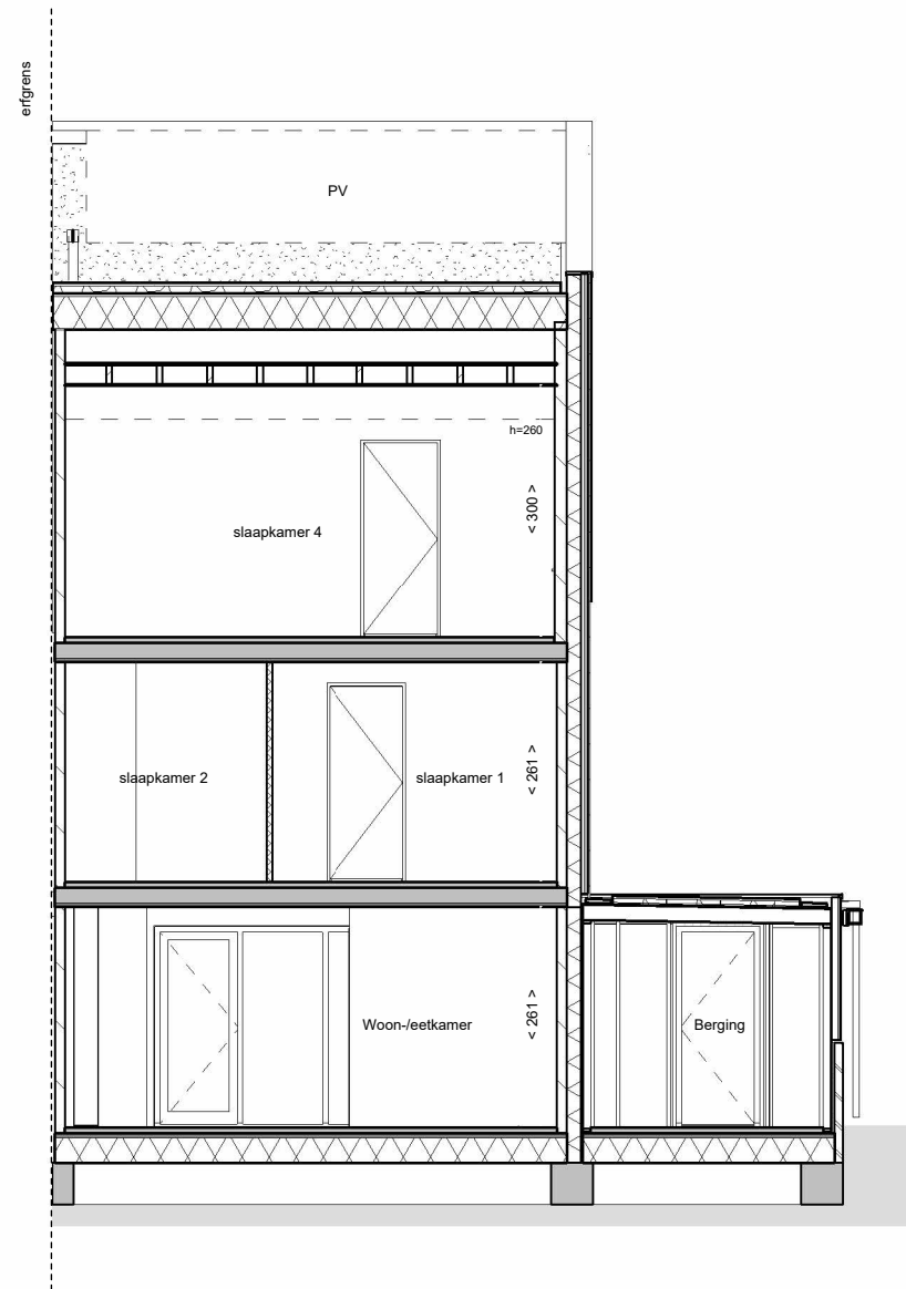
doorsnede A
