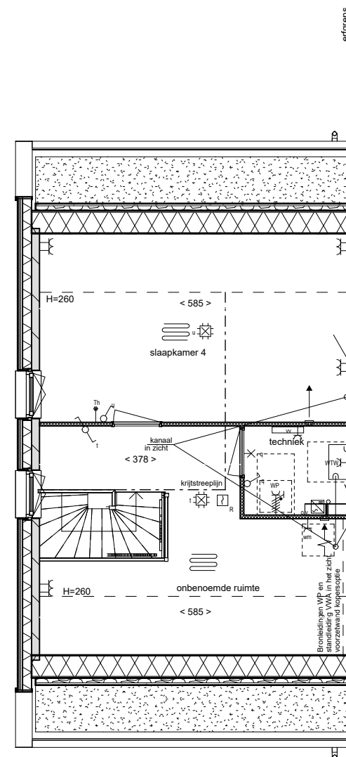
02 tweede verdieping
