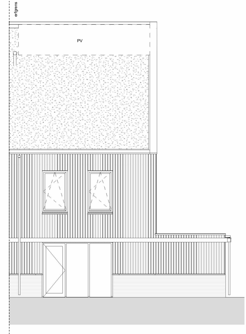
VK - bnr. 94 - achtergevel
