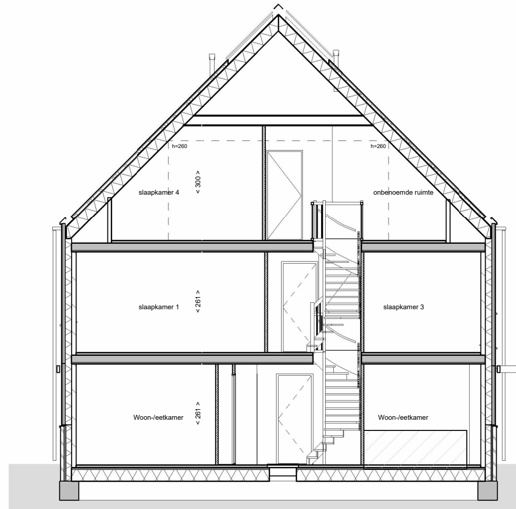
doorsnede B
