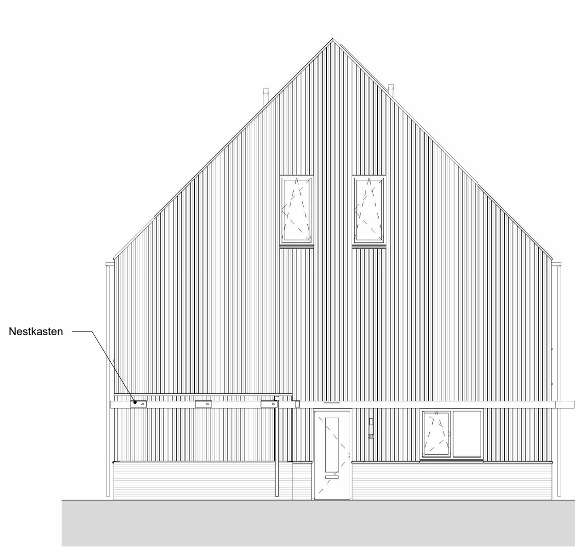
VK - bnr. 94 - zijgevel
