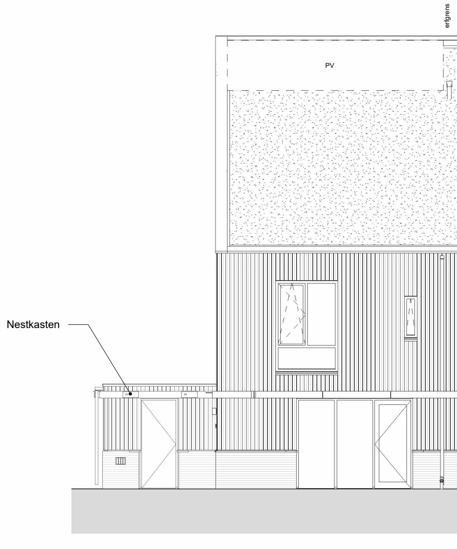
VK - bnr. 94 - voorgevel
