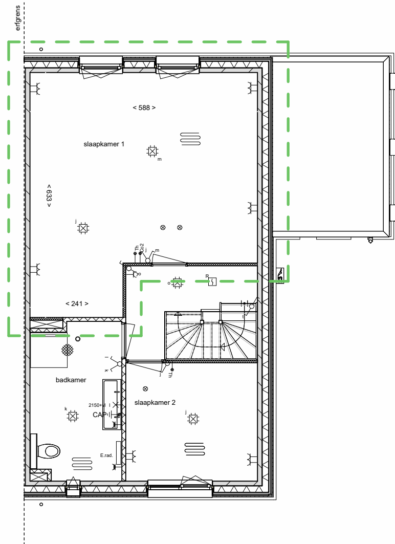
eerste verdieping
